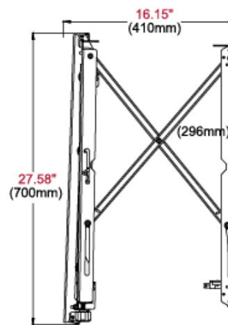
VUE LATÉRALE CONTRACTÉE
