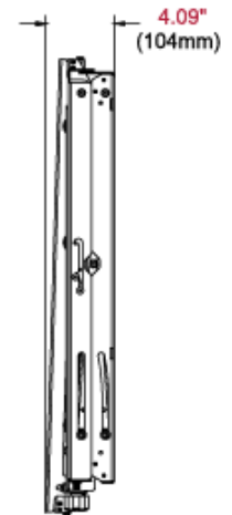
VUE LATÉRALE DÉPLOYÉE
